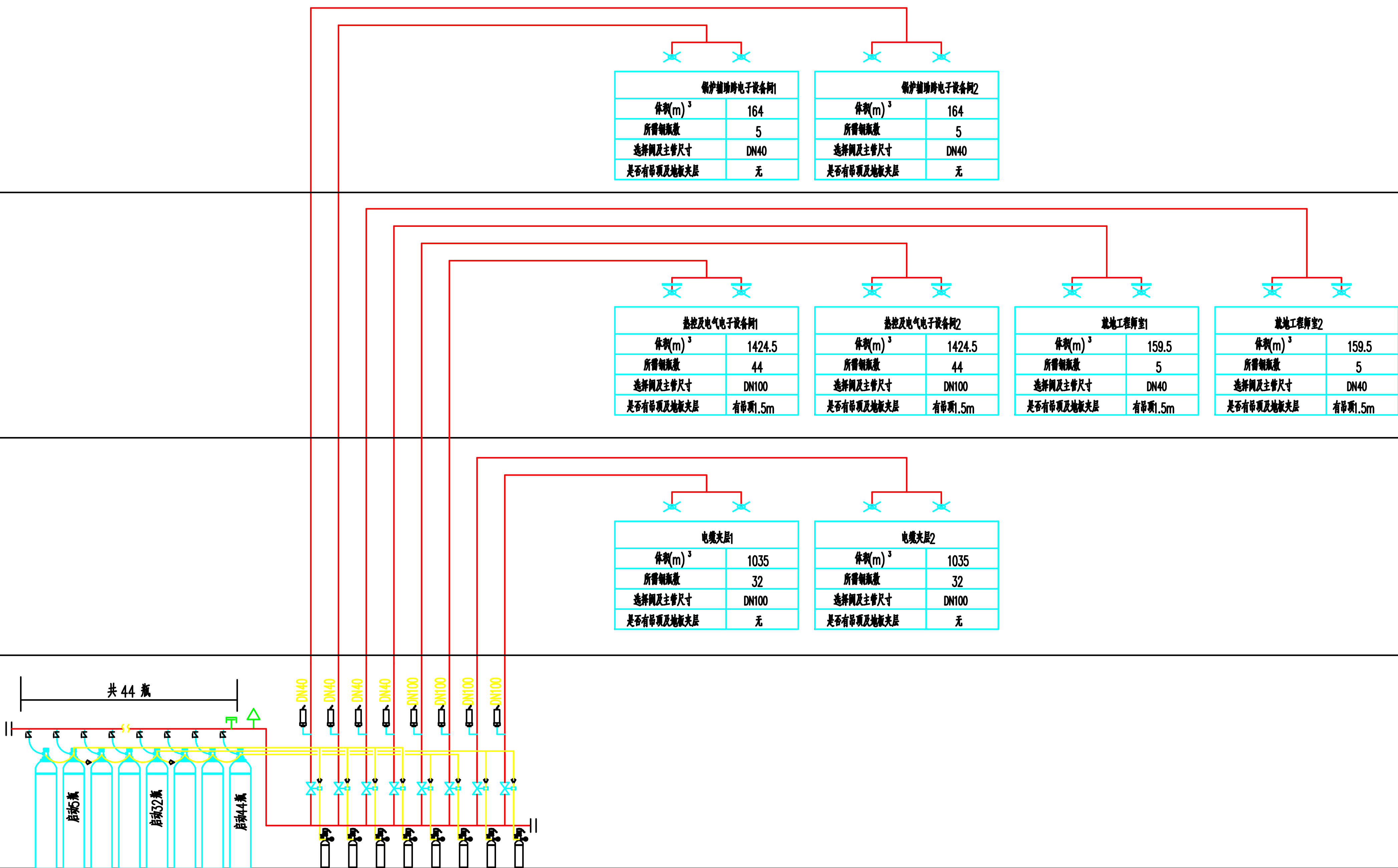
主厂房G541气体灭火原理图一
