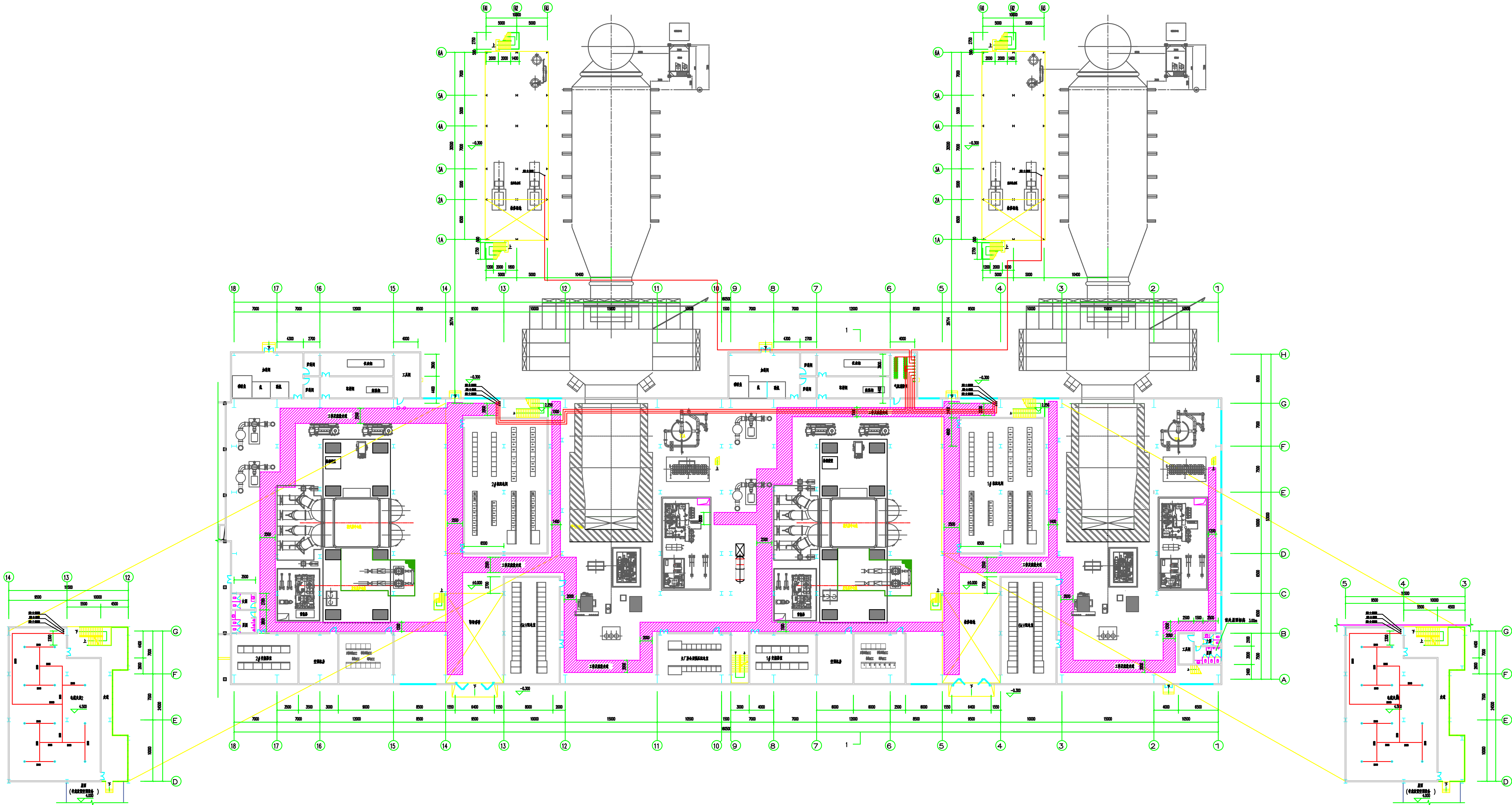
电缆夹层 4.500m 层平面图 1:200
